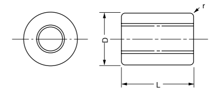
SNM型ストレートナット寸法表
