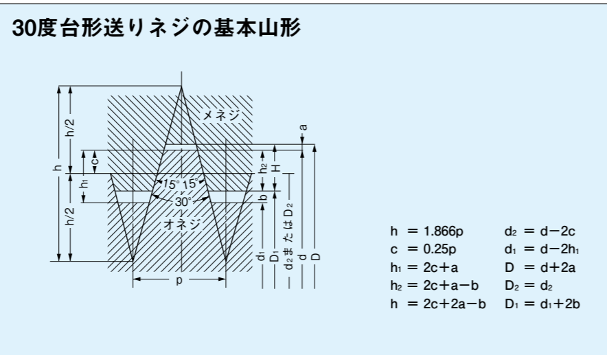
30度台形ネジ基本寸法
